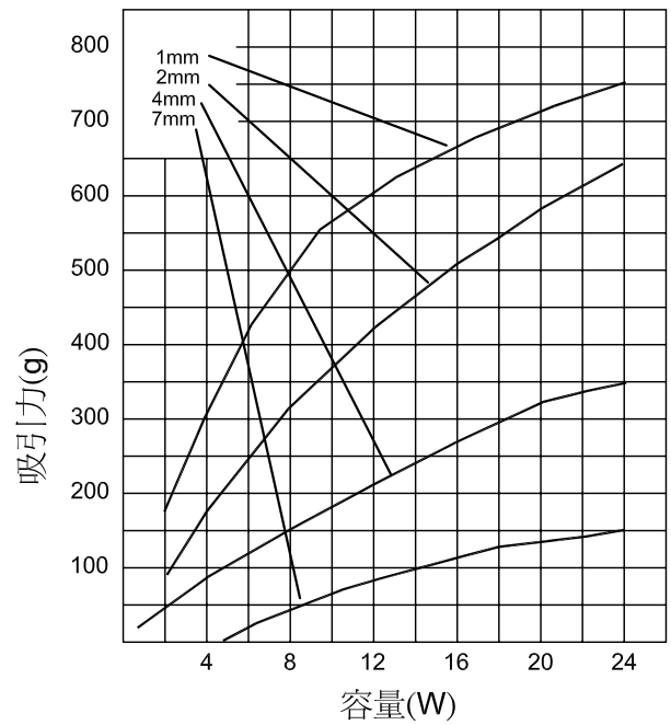
容量 / 吸引力
