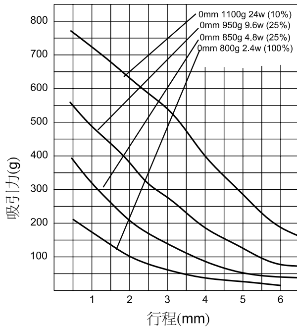
行程 / 吸引力
